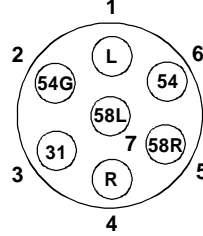
Perävaunun pistotulppa
