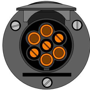
Perävaunu pistorasia
