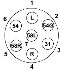
Perävaunu pistorasia
