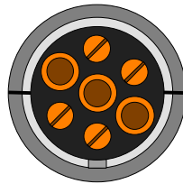
Perävaunun pistotulppa
